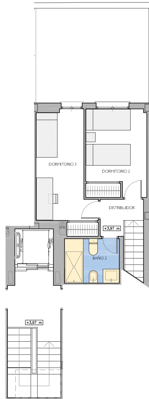
PLANTA ALTA
